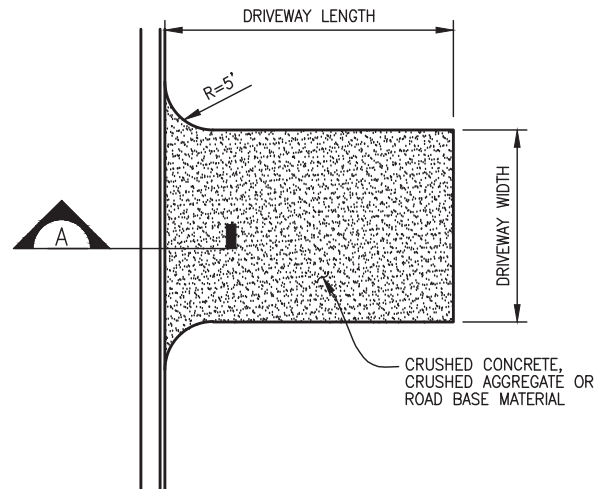
PLAN SCALE: 1" = 10'-0"
