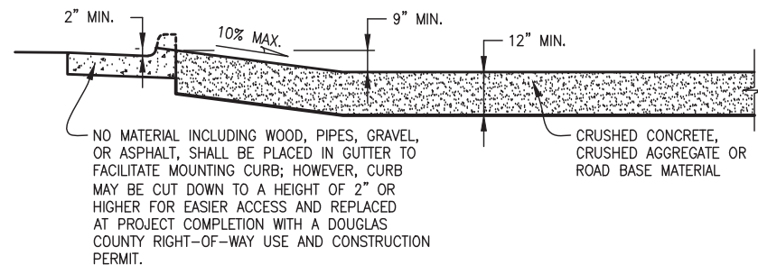
SECTION SCALE: 1/2" = 1'-0"
